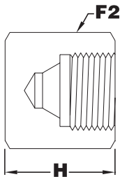
Blank Cap CGA 580
